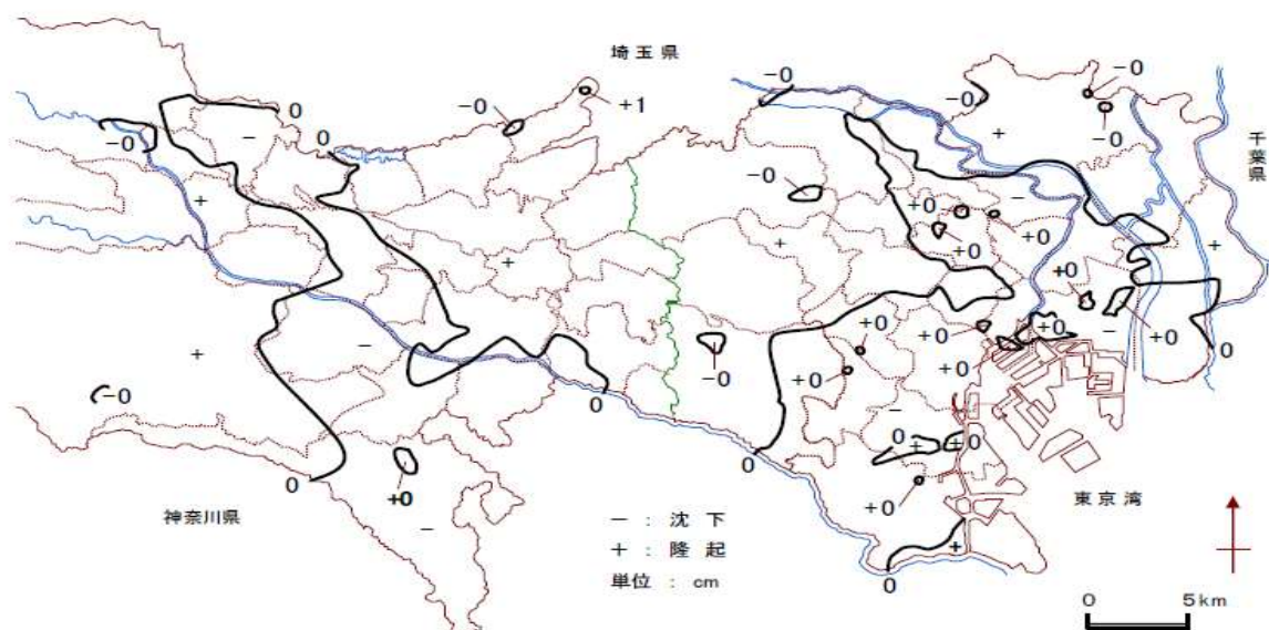
図－2 平成29年の地盤変動量図
