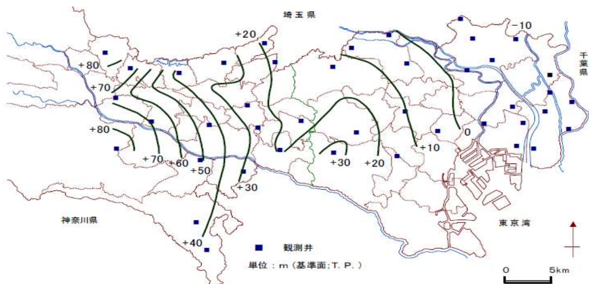
図－4 平成29年末の地下水位等高線図
