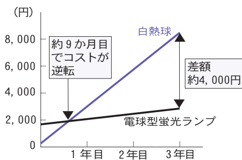
電球型蛍光灯と白熱球とのランニングコストの比較
