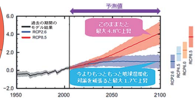
■ 出典 AR5 WG1 政策決定者向け要約 Fig SPM. 7(a)、Fig SPM. 8(a)
