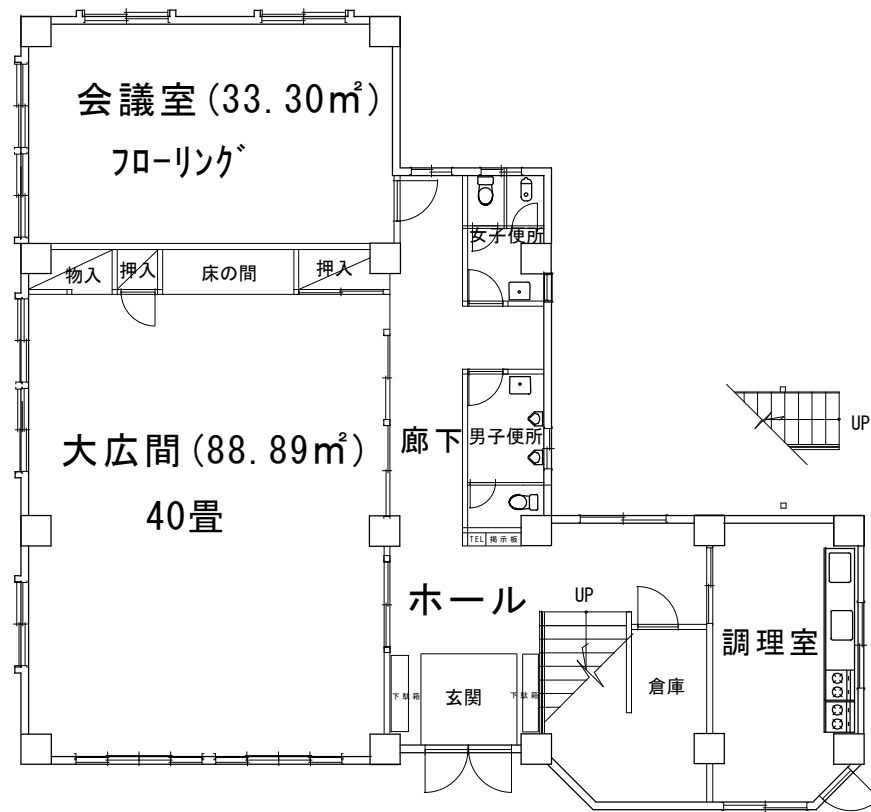
1 階平面図
