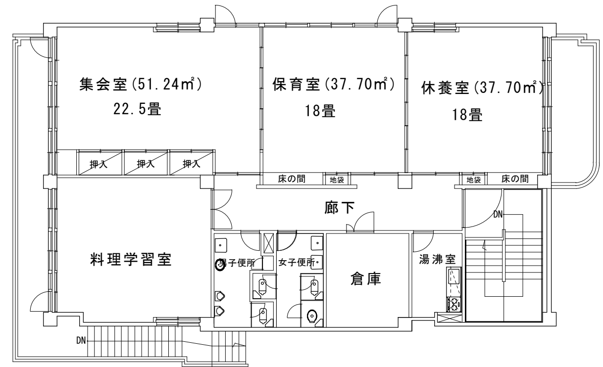
2階平面図
