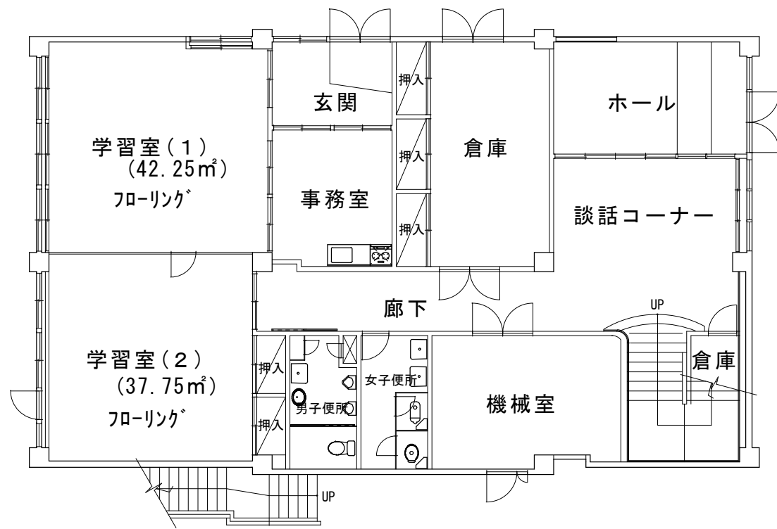
1階平面図
