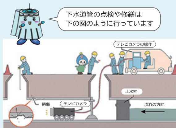
▲テレビカメラによる管路の調査などを行っています。
