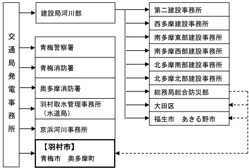
【白丸ダム放流通報情報伝達系統図】
