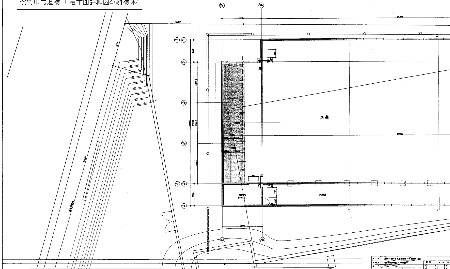
羽村市弓道場 1 階平面詳細図2(射場棟)
