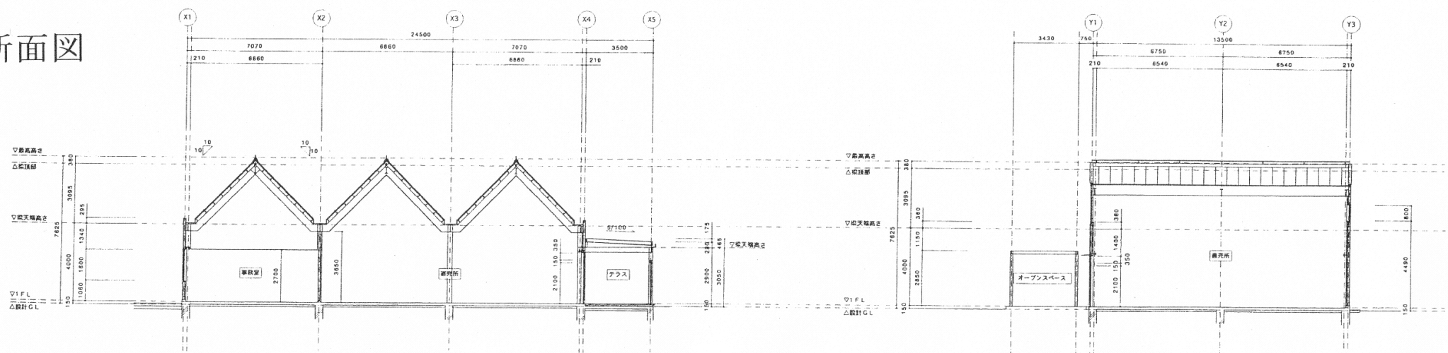
A-A 断面图
